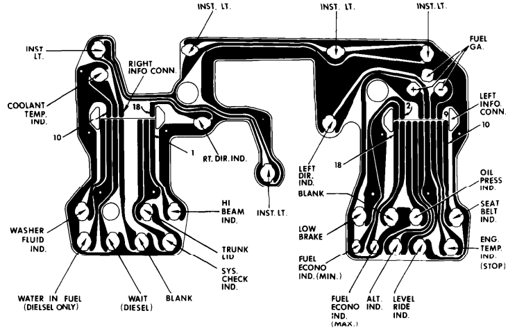
ELDORADO & SEVILLE P.C.
