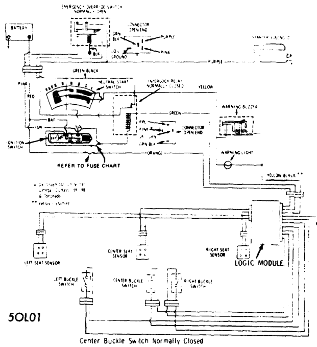
OLDSMOBILE STARTER INTERLOCK WIRING
