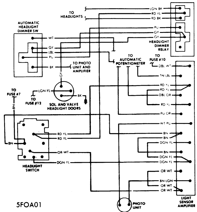
FORD MOTOR CO. AUTOLAMP.
