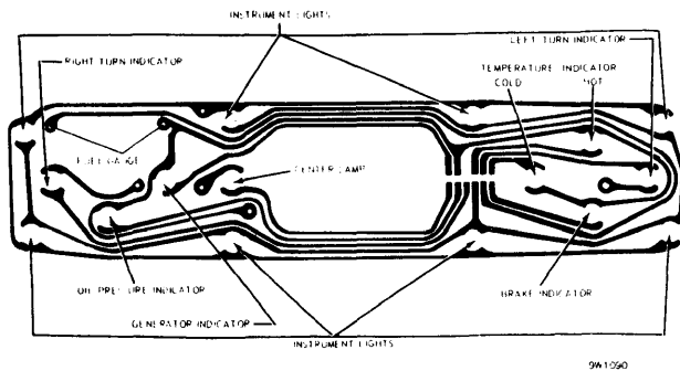
1969-70 (EXC. F-85 & TORONADO)
