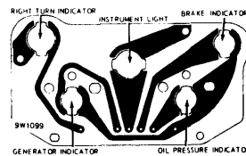
1968-70 TORONADO (GEN. & OIL)
