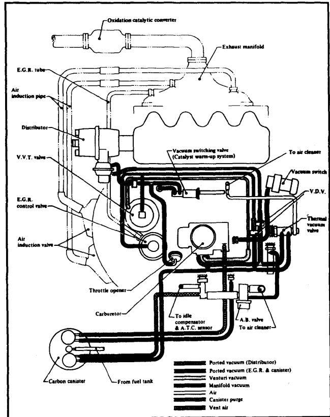
Fig. 8: Datsun Sentra Exc. M.P.G. & 310 (Federal)
