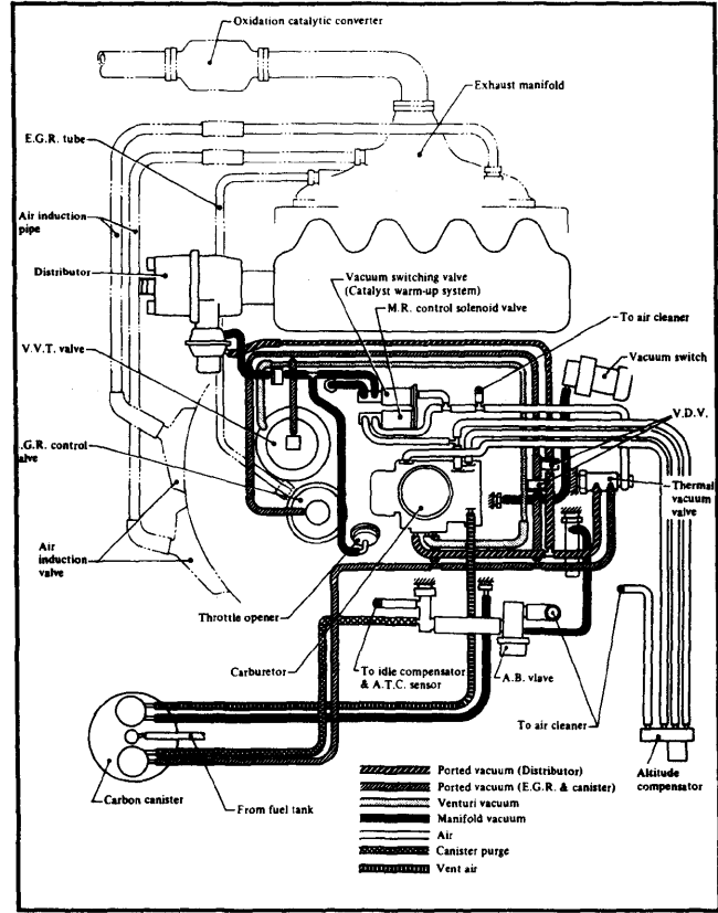
Fig. 7: Datsun Sentra Exc. M.P.G. & 310 (California)
