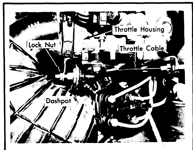
Fig. 1 Saab Dashpot
