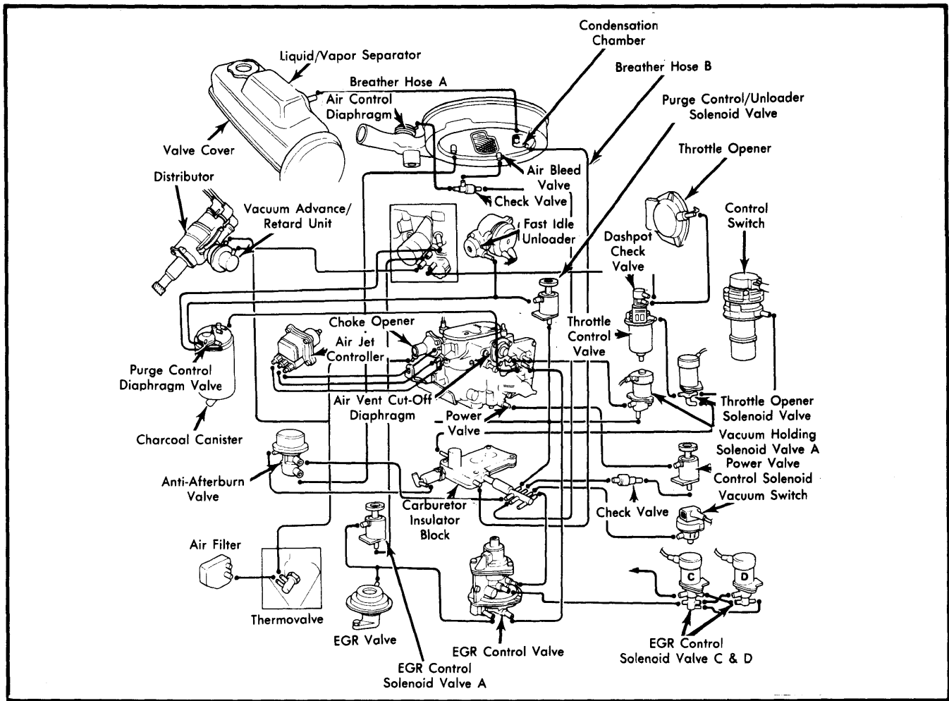
Fig. 7 Accord & Prelude Calif. Auto. Trans.
