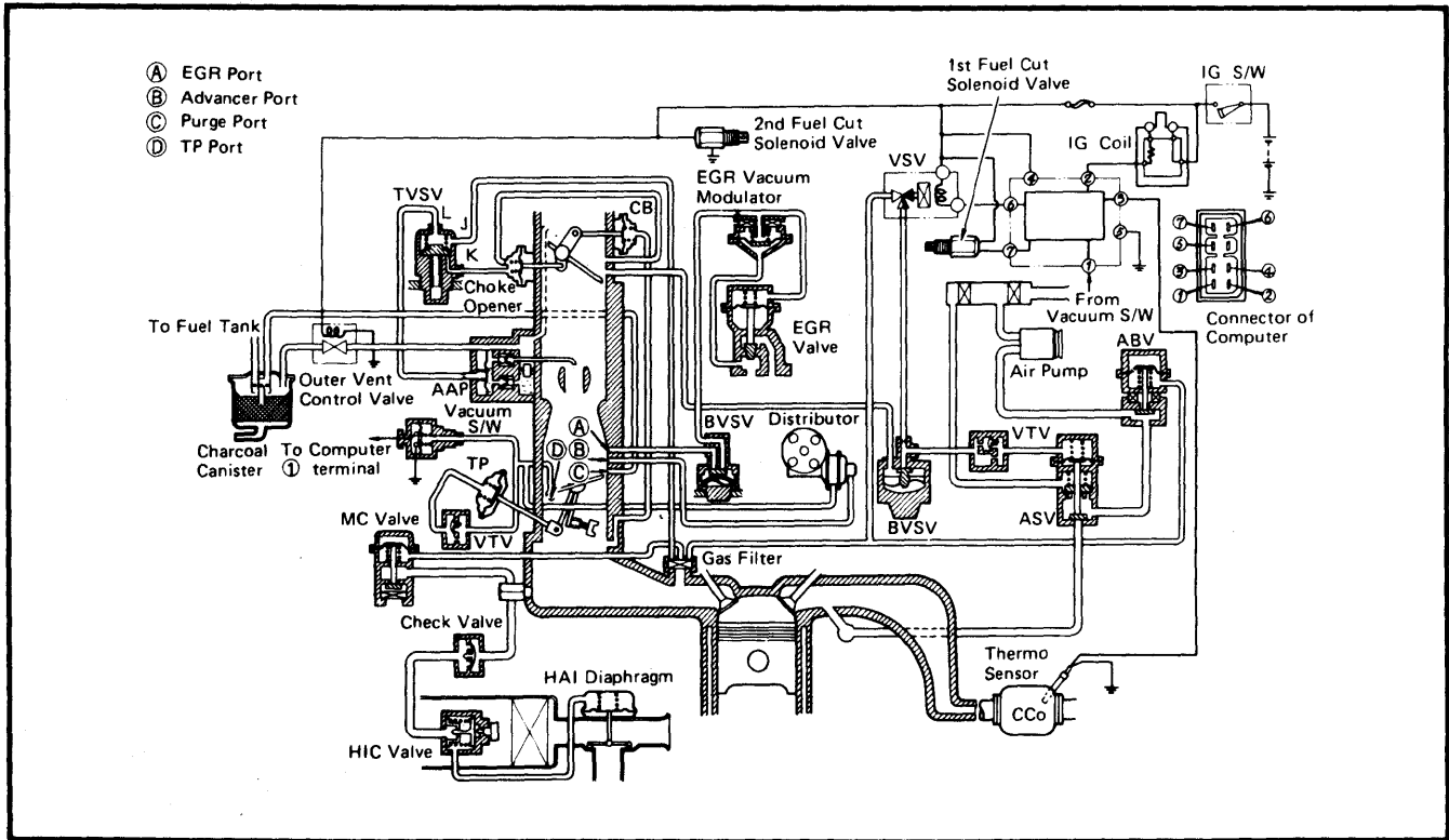
Fig. 5 Toyota Corolla (California)
