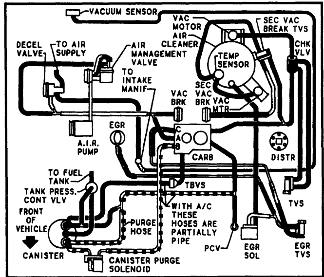
Fig. 8 2.8L (173") V6 2-Bbl. VIN X Federal, Calif. Auto. & Man. Trans.
