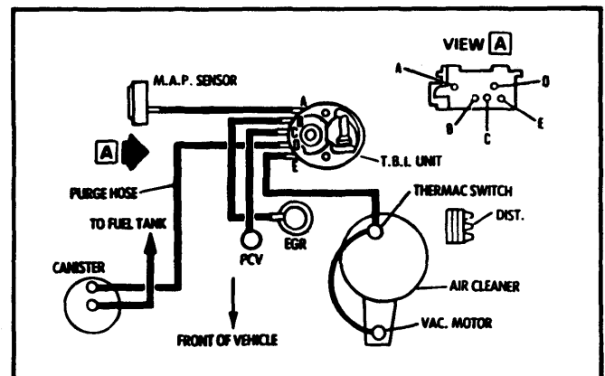
Fig. 4 1.8L (112") 4 Cyl. EFI, VIN O Federal Auto. & Man. Trans.
