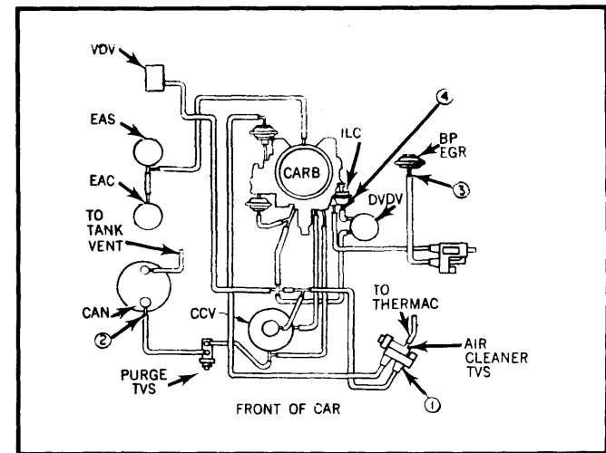
Fig. 18 5.0L (307'') V8 4-Bbl. VIN Y Calif. Auto. Trans.
