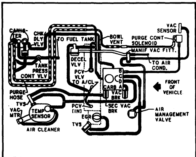
Fig. 5 2.0L (122") 4 Cyl. 2-Bbl. Hi. Alt. Auto. Trans.
