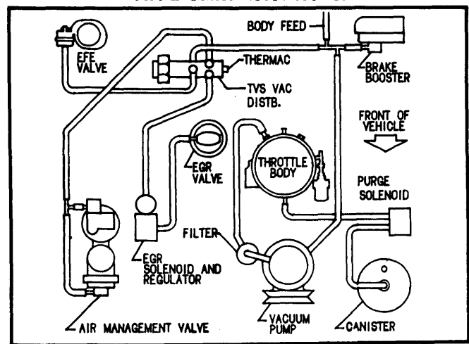
Fig. 12 4.1L (250") V8 DFI VIN 8 All Auto. Trans.
