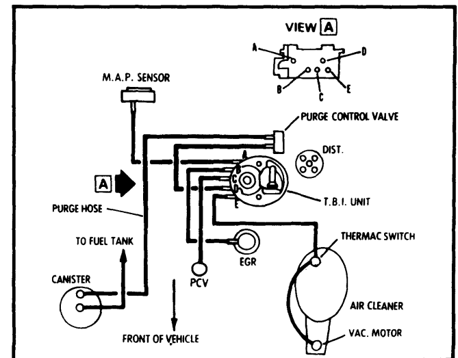
Fig. 6 2.5L (151") 4 Cyl. EFI, VIN R Hi. Alt. Auto. & Man. Trans.
