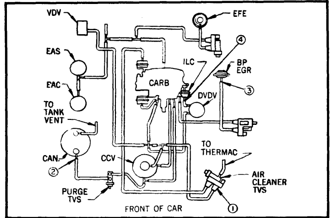
Fig. 14 4.3L (260'') V8 2-Bbl. VIN 8 Federal Auto. Trans.
