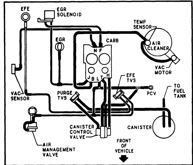
Fig. 16 5.0L (305'') V8 4-Bbl. VIN H Federal, Calif. Auto. Trans.
