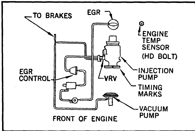
Fig. 13 4.3L (262'') V6 Diesel VIN V Federal Auto. Trans.
