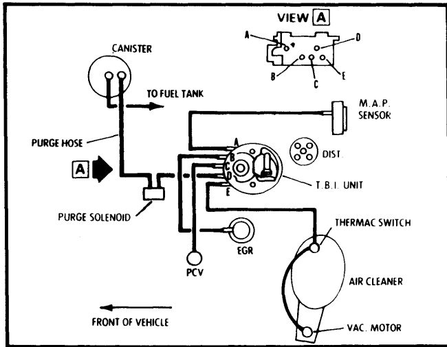
Fig. 7 2.5L (151") 4 Cyl. 2-Bbl. VIN 2 Hi. Alt. Auto. & Man. Trans.
