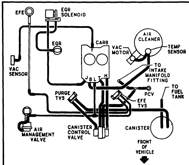
Fig. 15 4.4L (267'') V8 2-Bbl. VIN J Federal Auto. Trans.
