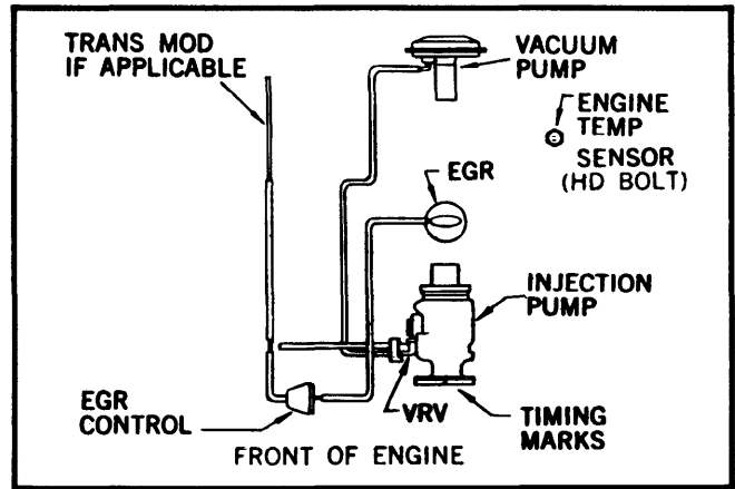
Fig. 20 5.7L (350") V8 Diesel VIN N Hi. Alt. Auto. Trans.
