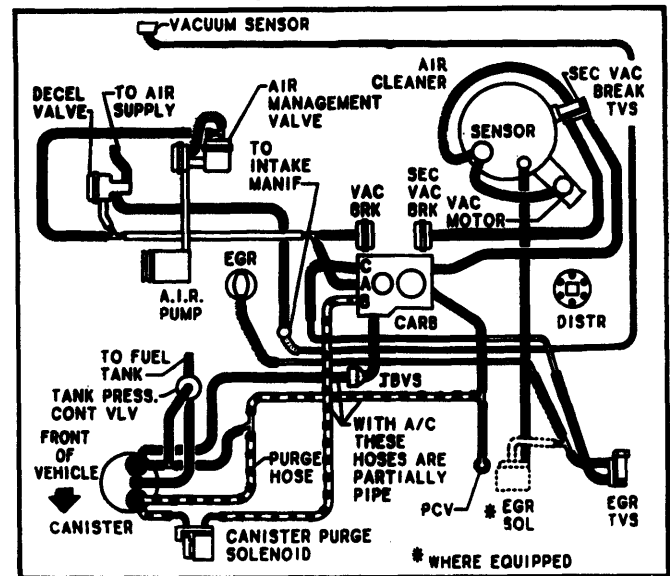
Fig. 10 2.8L (173") V6 2-Bbl. VIN Z Calif. Auto. Trans.
