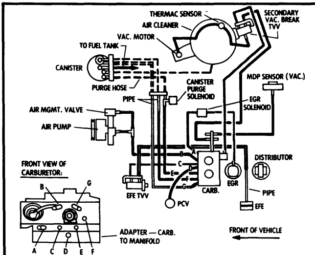
Fig. 20 4.3L (265") V8 All Models
