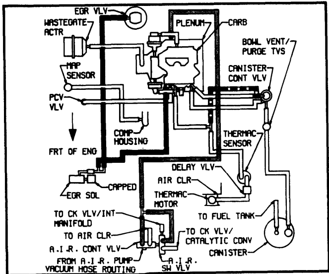
Fig. 16 3.8L (231") Turbo V6 Calif. Auto. Trans.
