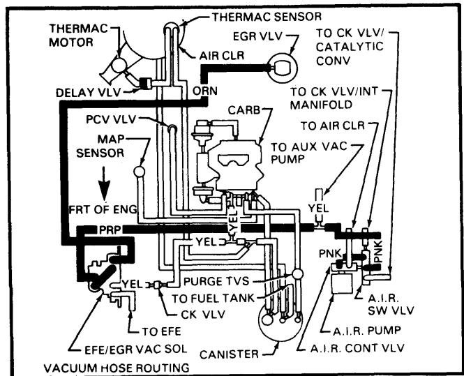
Fig. 18 4.1L (252") V6 Calif. Auto. Trans.
