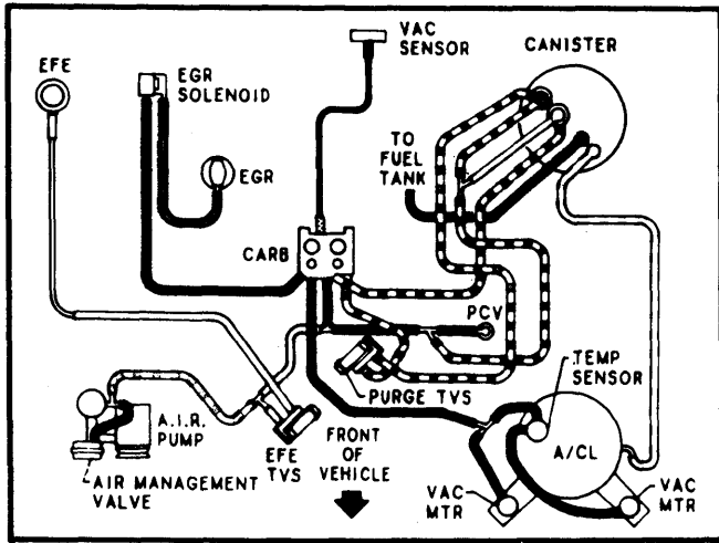
Fig. 25 5.7L (350") V8 Calif.
