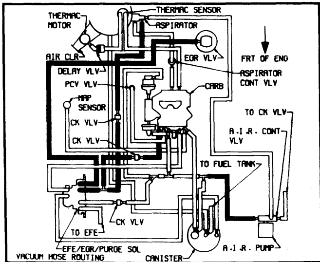
Fig. 14 3.8L (231") V6 Calif. Auto. Trans.
