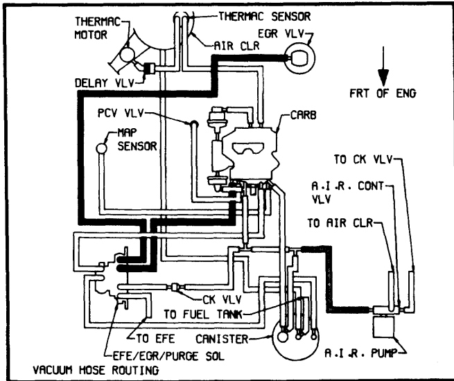
Fig. 13 3.8L (231") V6 Calif. Auto. Trans.
