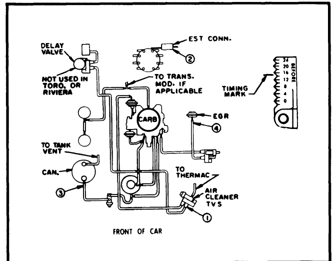
Fig. 23 5.0L (307") V8 All Models
