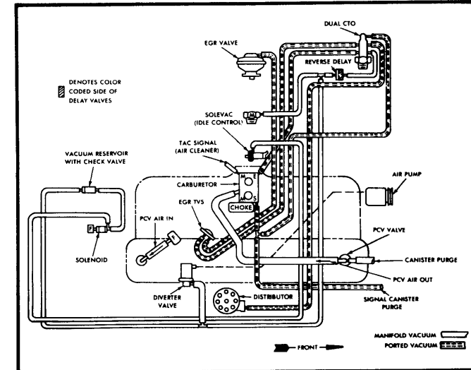
Fig. 12 258" 6 Cyl. High Altitude – Eagle (Auto. Trans.)
