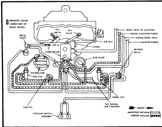
Fig. 8 151" 4 Cyl. Calif. – Eagle (Auto. Trans.)
