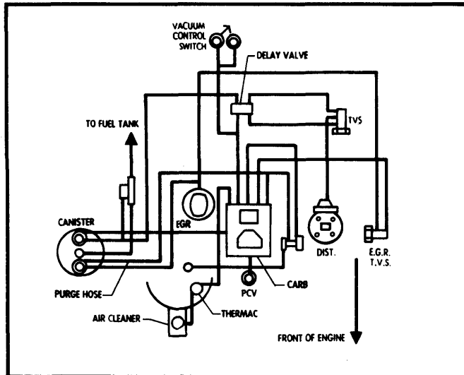
Fig. 14 151" 4 Cyl. 2-Bbl. VIN 5 Calif. Man. Trans.
