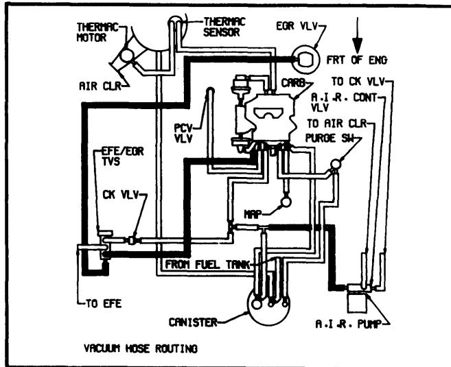
Fig. 31 231" V6 2-Bbl. Calif. Auto. Trans.
