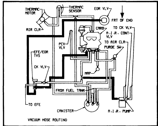
Fig. 29 231" V6 2-Bbl. Calif. Auto. Trans.
