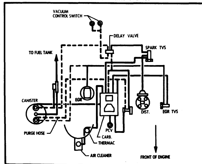
Fig. 15 151" 4 Cyl. 2-Bbl. VIN 5 Calif. Auto. Trans.
