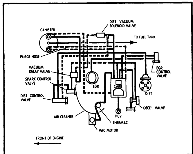
Fig. 6 151" 4 Cyl. 2-Bbl. VIN V Federal
