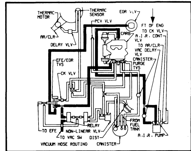
Fig. 60 350" V8 4-Bbl. VIN X Federal Auto. Trans.
