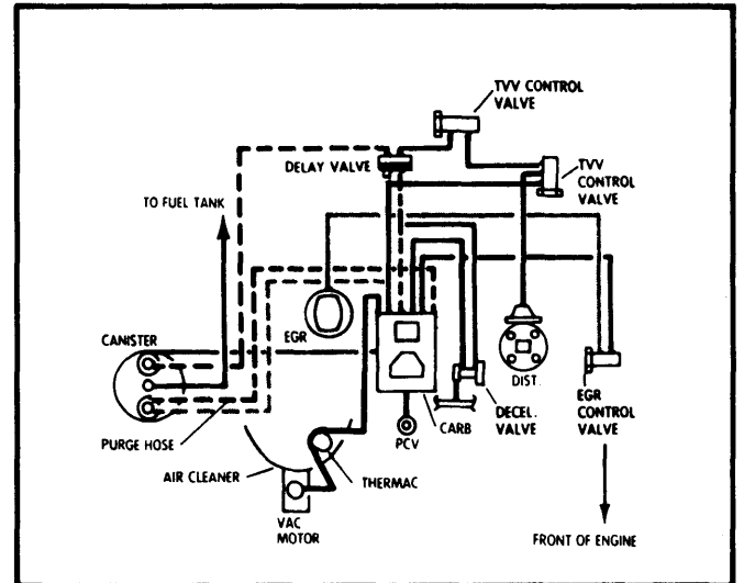
Fig. 11 151" 4 Cyl. 2-Bbl. VIN 5 Federal Auto. Trans.
