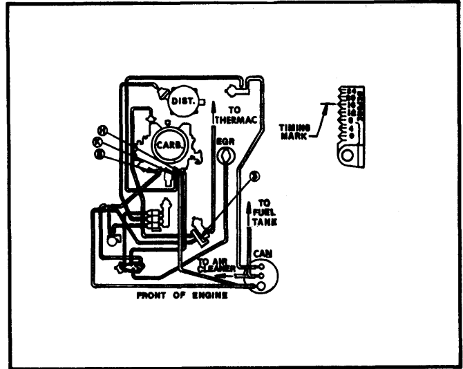
Fig. 58 350" V8 4-Bbl. VIN R Calif. Auto. Trans.
