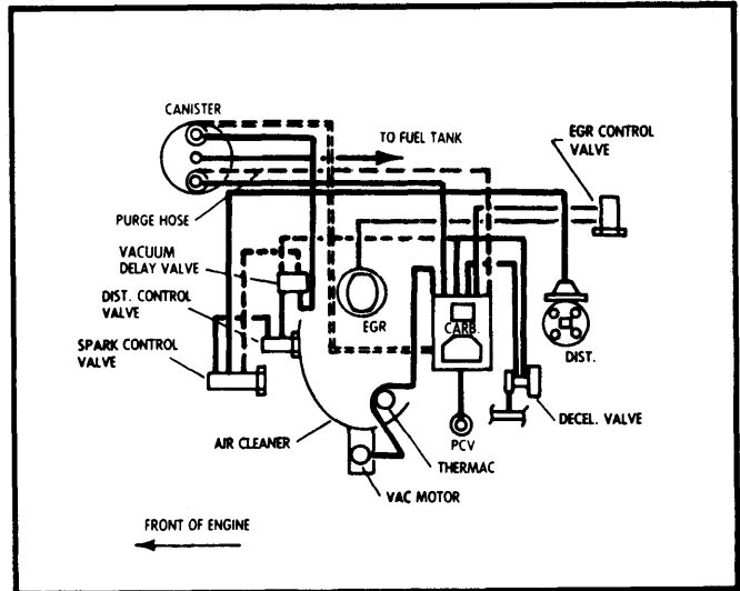
Fig. 5 151" 4 Cyl. 2-Bbl. VIN V Federal
