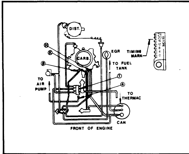
Fig. 56 350" V8 4-Bbl. VIN R Federal Auto. Trans.
