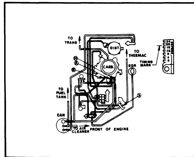
Fig. 57 350" V8 4-Bbl. VIN R Calif. Auto. Trans.
