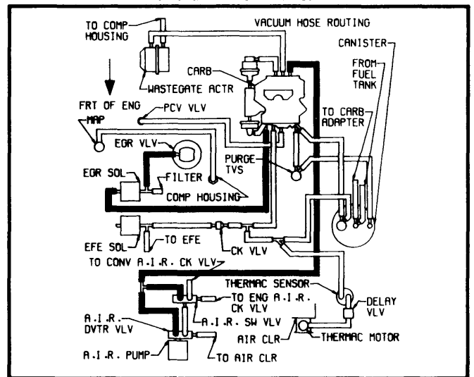
Fig. 35 231" V6 Turbo Calif. Auto. Trans.
