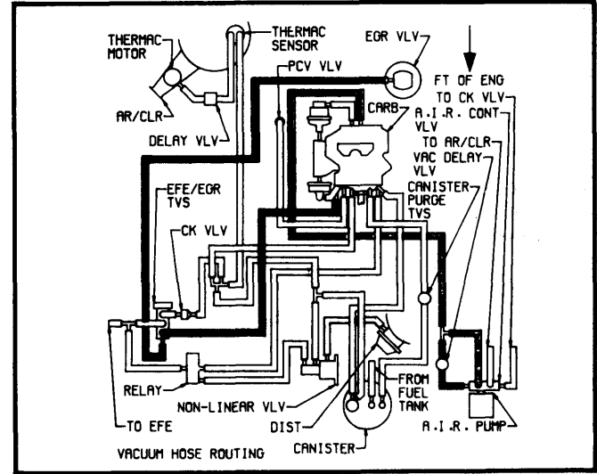
Fig. 59 350" V8 4-Bbl. VIN X Federal Auto. Trans.
