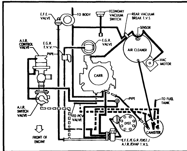
Fig. 65 368" V8 4-Bbl. Calif. Auto. Trans.
