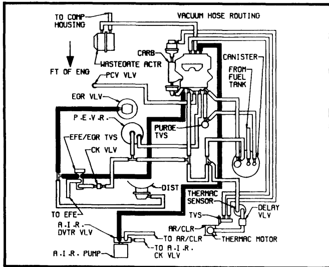
Fig. 32 231" V6 Turbo Federal Auto. Trans.
