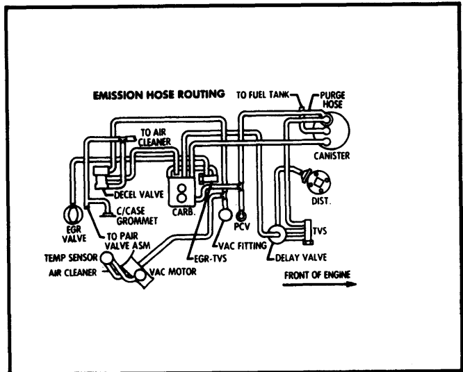
Fig. 4 98" 4 Cyl. 2-Bbl. Calif.
