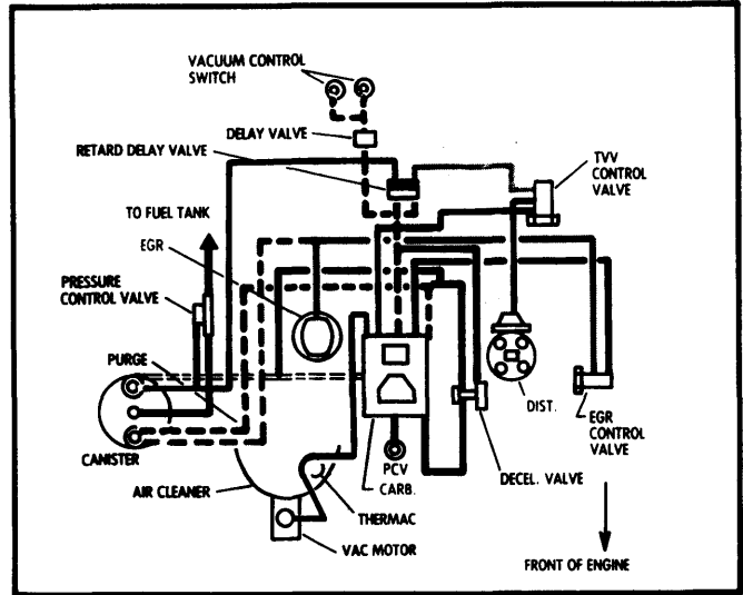
Fig. 16 151" 4 Cyl. 2-Bbl. VIN 5 Calif. Auto. Trans.
