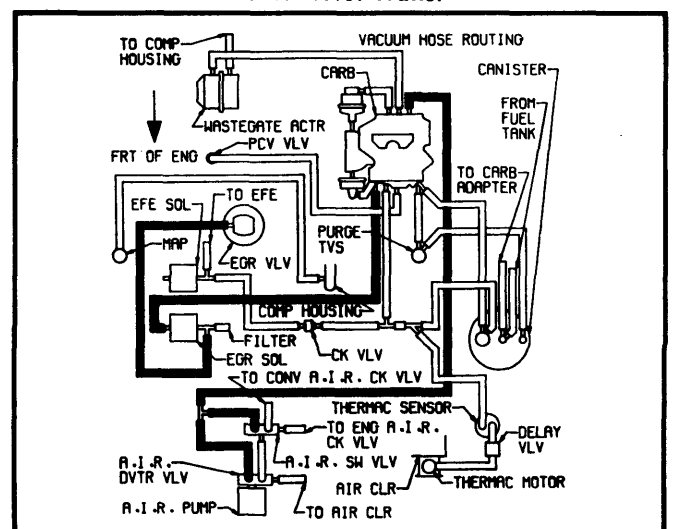
Fig. 36 231" V6 Turbo Calif. Auto. Trans.
