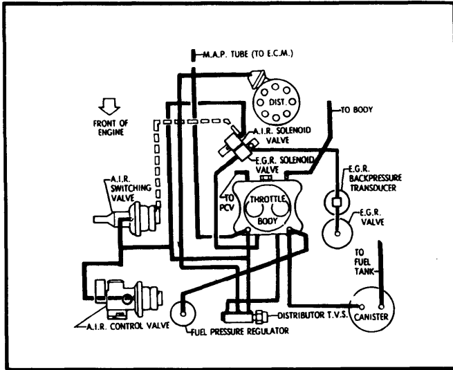
Fig. 61 350" V8 EFI Calif. Auto. Trans.
