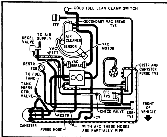
Fig. 19 173" V6 2-Bbl. Calif. Auto. Trans.
