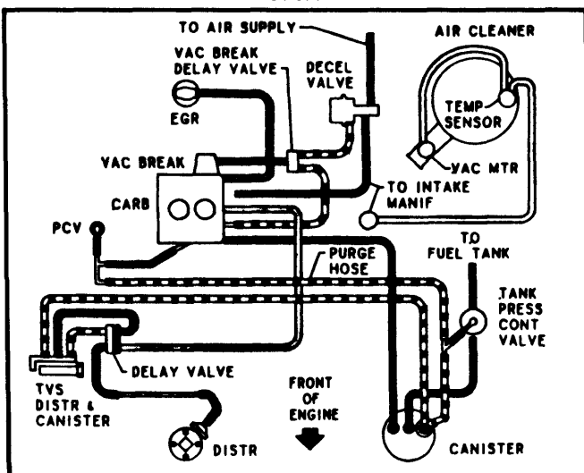
Fig. 3 98" 4 Cyl. 2-Bbl. Calif.
