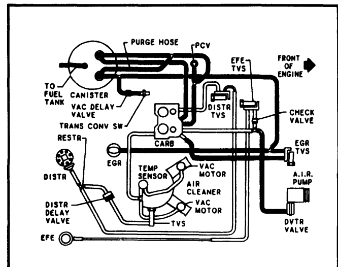
Fig. 54 350" V8 4-Bbl. VIN 6 & 8 Federal Auto. Trans.
