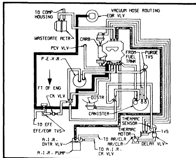
Fig. 33 231" V6 Turbo Federal Auto. Trans.
