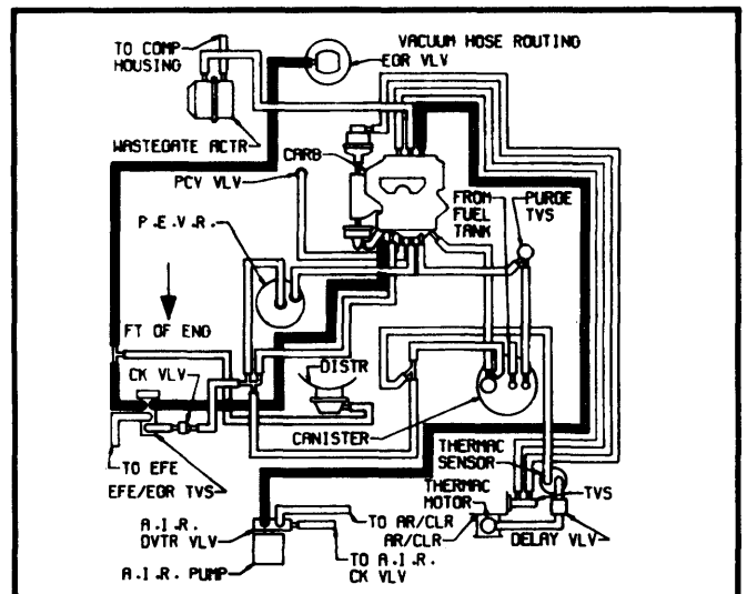
Fig. 34 231" V6 Turbo Federal Auto. Trans.
