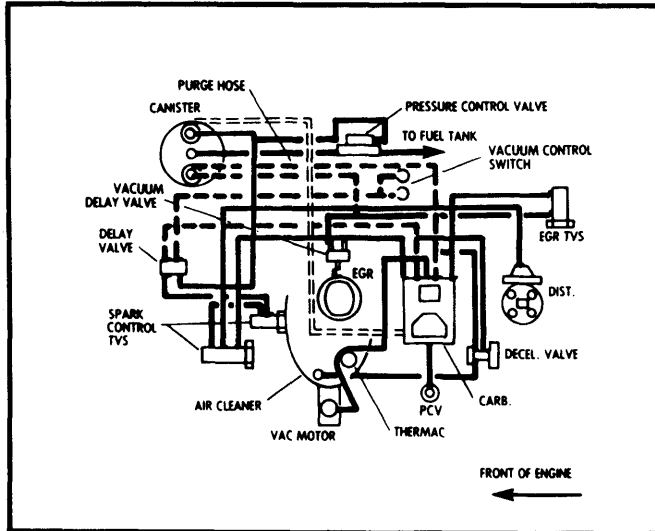
Fig. 8 151" 4 Cyl. 2-Bbl. VIN V Calif. Auto. Trans.
