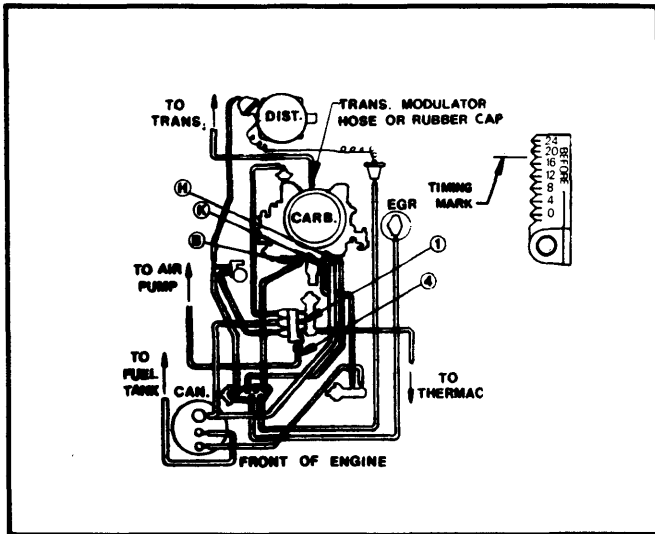
Fig. 55 350" V8 4-Bbl. VIN R Federal Auto. Trans.
