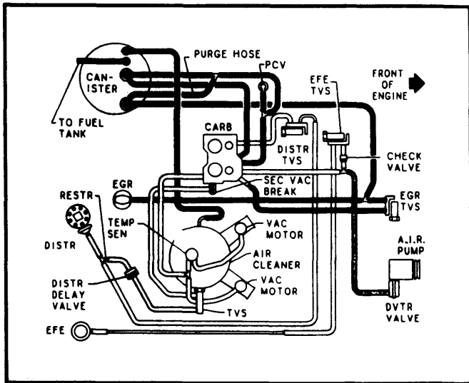
Fig. 49 305" V8 4-Bbl. Calif. Auto. Trans.
