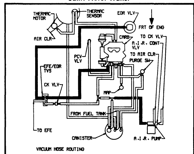
Fig. 30 231" V6 2-Bbl. Calif. Auto. Trans.
