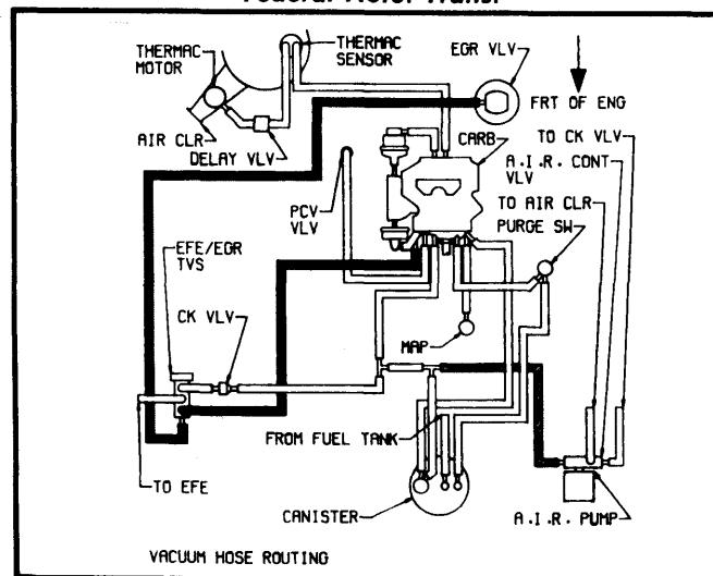
Fig. 27 231" V6 2-Bbl. Federal Auto. Trans. W/C-A
