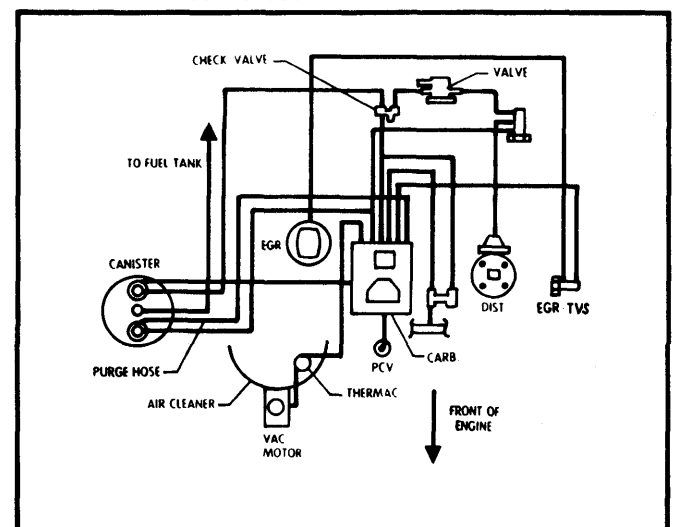
Fig. 12 151" 4 Cyl. 2-Bbl. VIN 5 Federal Auto. Trans.
