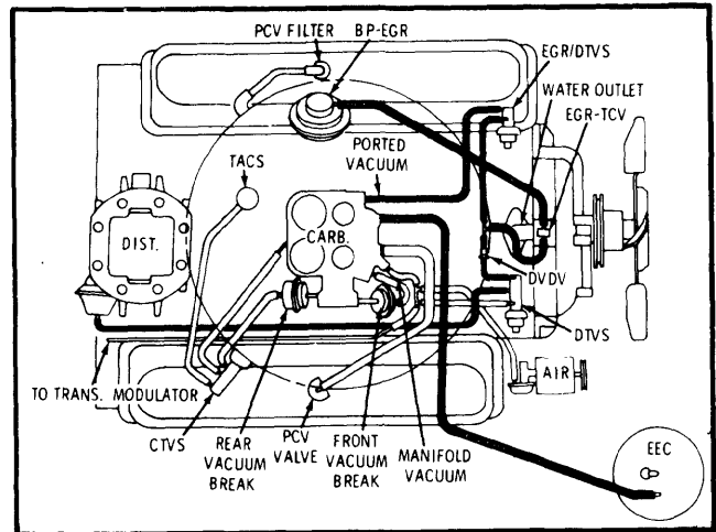
Fig. 14 350 CID VIN "R" & 403 CID Vac. Hose Routing (Calif.)
