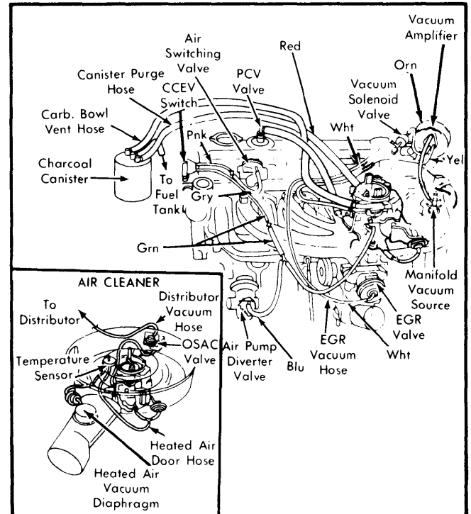
Fig. 4 225" 1-Barrel; California; Auto. Trans.
