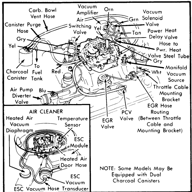
Fig. 8 318" 4-Barrel; California; Auto. Trans.
