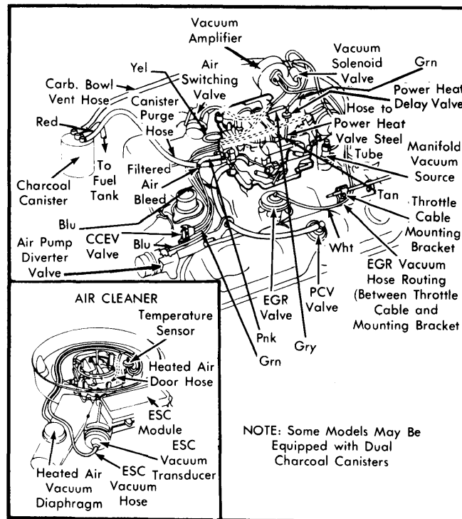
Fig. 11 360" 4-Barrel; California; Auto. Trans.
