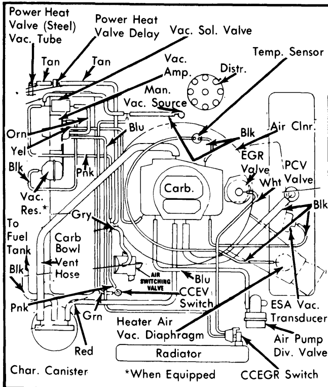
Fig. 7 318" 4-Bbl., Calif., Auto. Trans.
