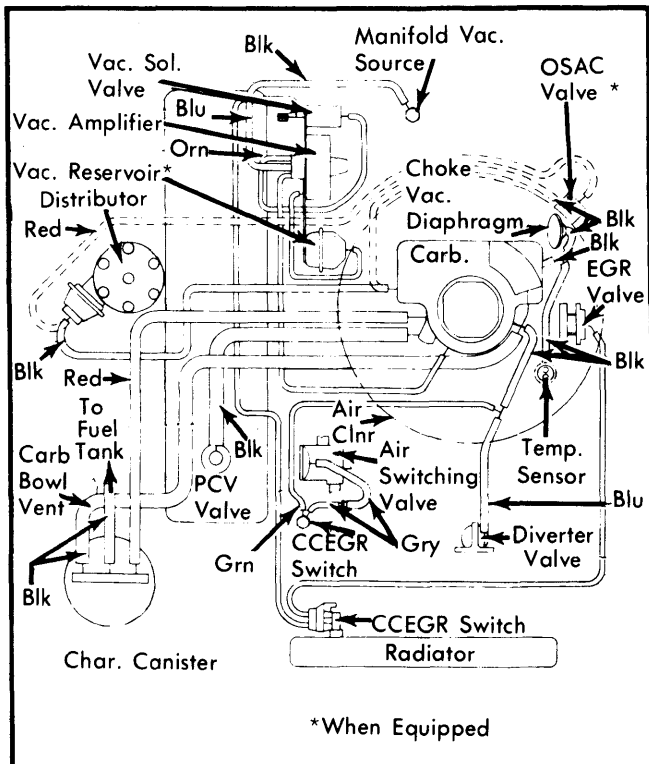
Fig. 3 225", High Alt. and Calif., Auto. Trans.
