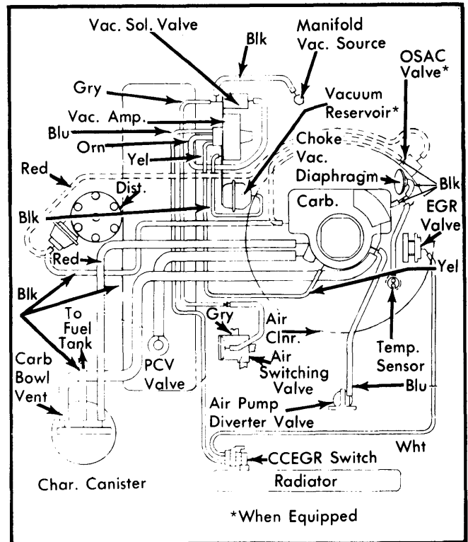
Fig. 4 225", Calif., Man. Trans.
