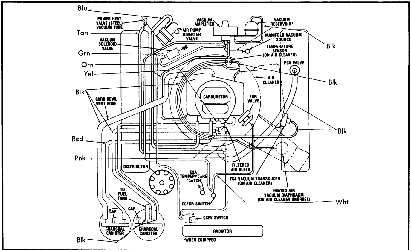
Fig. 19 440" 4-Bbl., High Alt. and Calif., Auto. Trans.
