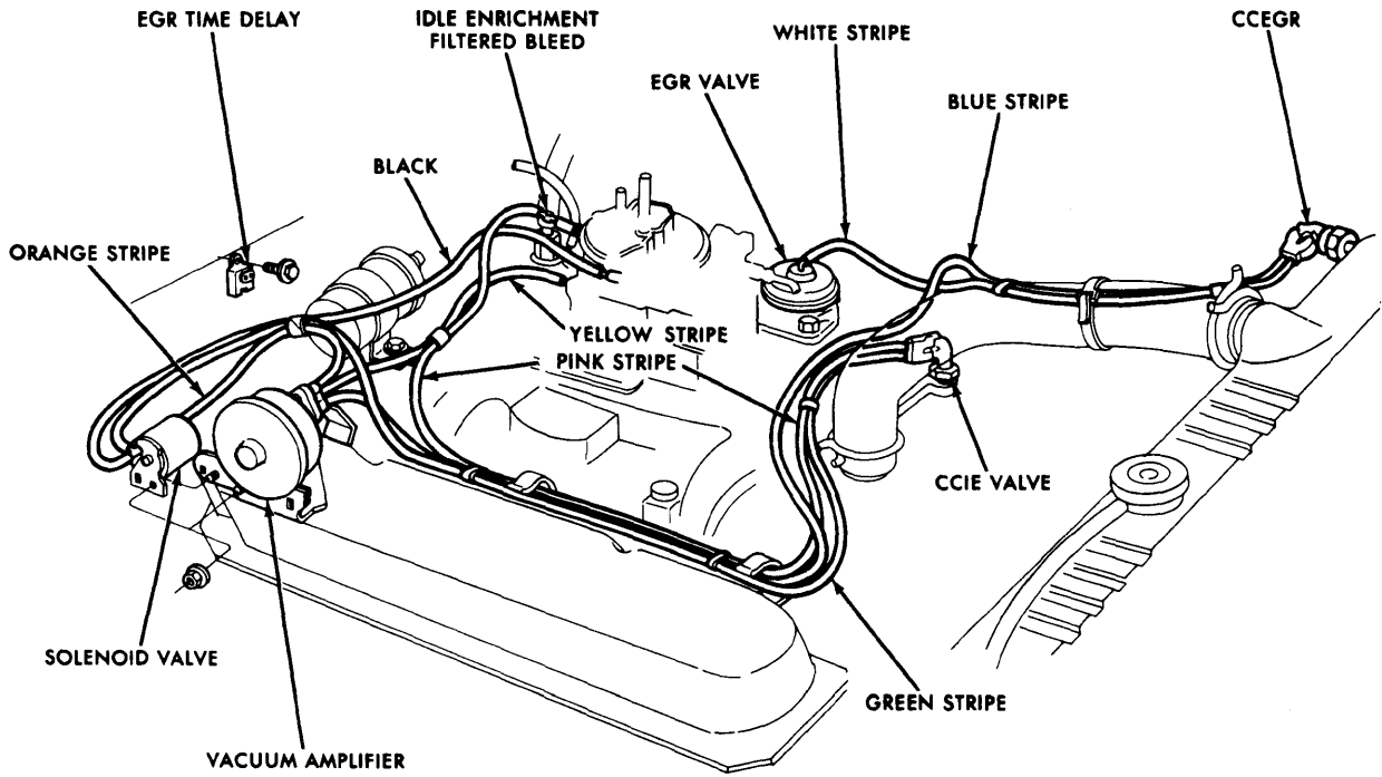
EGR SYSTEM 318" AUTO. TRANS. (CALIFORNIA)
