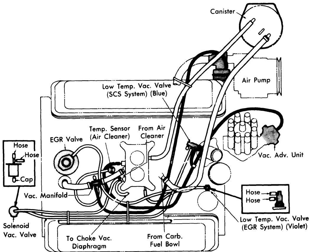
1974 IHC 400" V8
