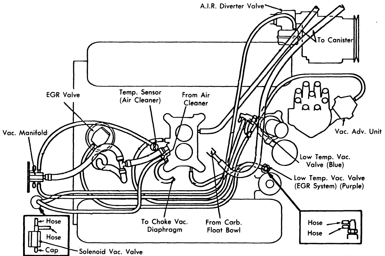
1973 IHC 400" V8
