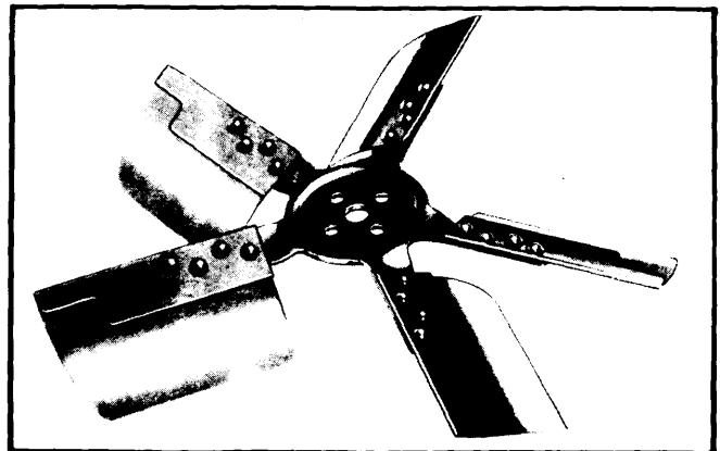
Fig. 2 Flex-Blade Fan
