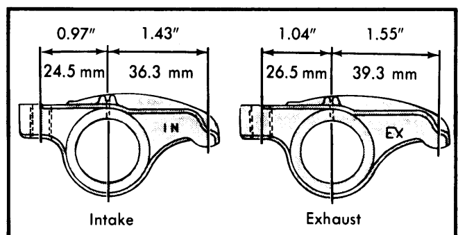
Fig. 7 Rocker Arms
