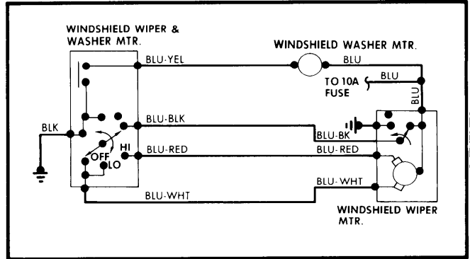
Fig. 4 Mazda B2000 Wiring Diagram
