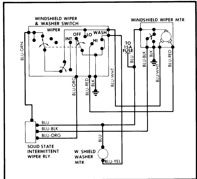
Fig. 5 Mazda 626 Wiring Diagram
