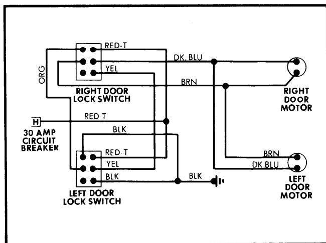
Fig. 1 AMC Door Lock Wiring Diagram
