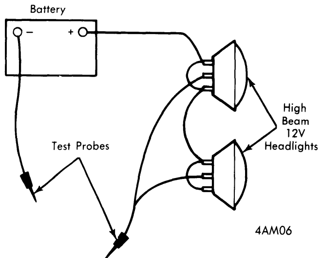
RECTIFIER DIODE LOAD TEST
