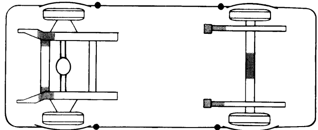
Renault
