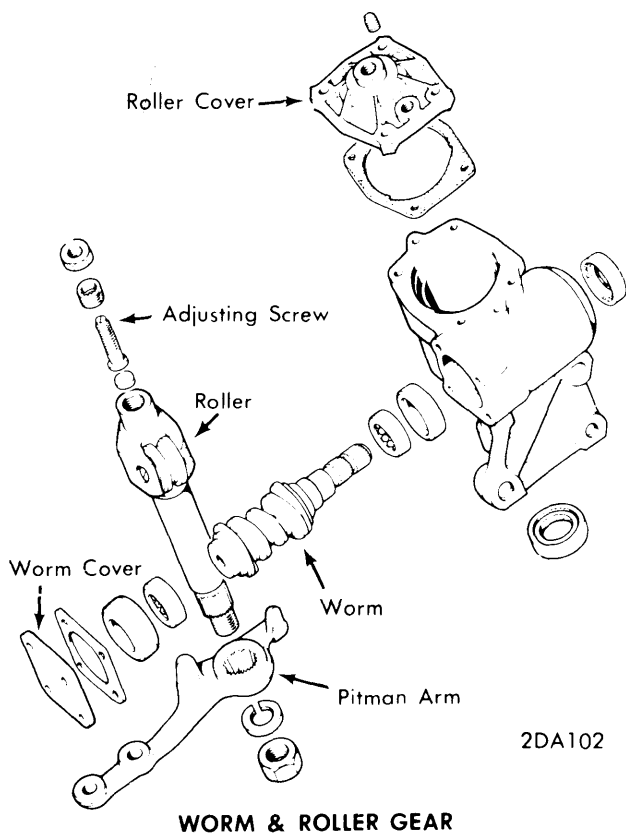
WORM & ROLLER GEAR
