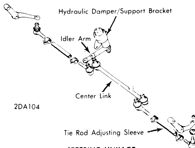
STEERING LINKAGE (124 COUPE & SPIDER)
