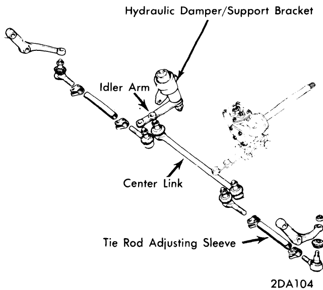
STEERING LINKAGE (124 COUPE & SPIDER)
